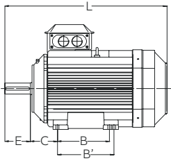
Foot-mounted motor IM 1001, IM B3
