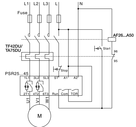
Sigortalar, kontaktör ve termik röle ile
