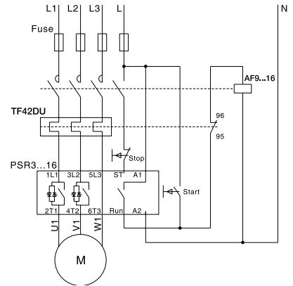
Sigortalar, kontaktör ve termik röle ile
