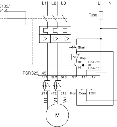
E) MKŞ ve yardımcı kontak ile
