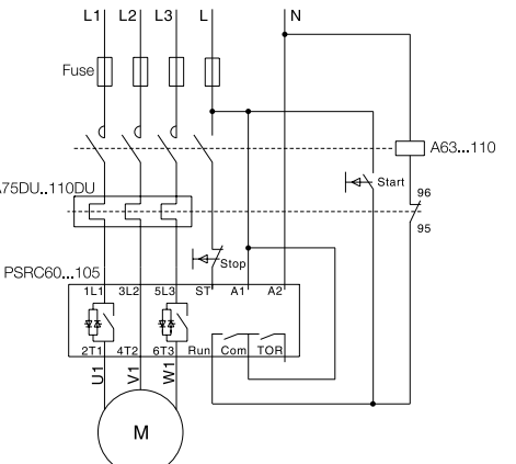
I) Sigortalar, kontaktör ve termik röle ile
