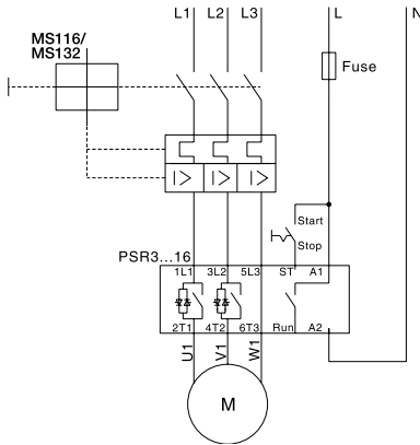
PSR3 ... PSR16 (MKŞ ile)
