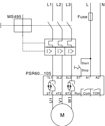
PSR60 ... PSR105 (MKŞ ile)
