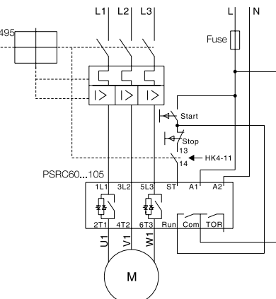
H) MKŞ ve yardımcı kontak ile
